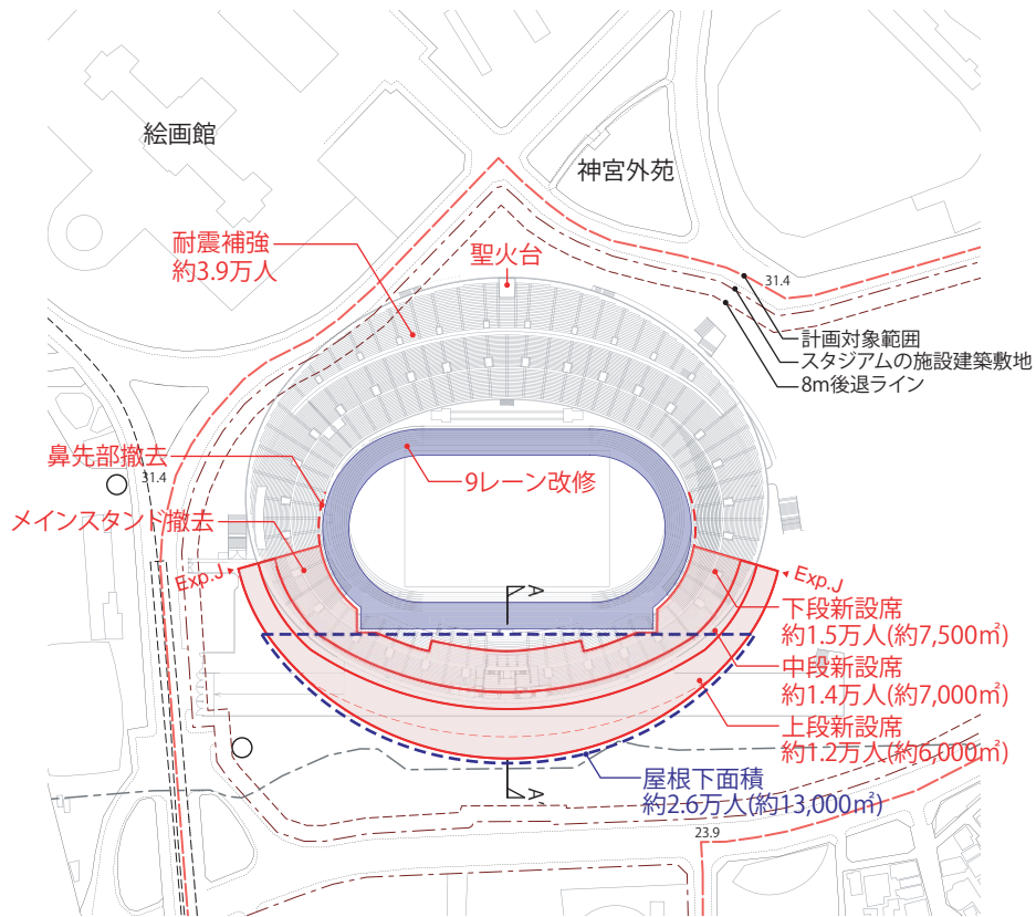
平面図 0 20 50 100(m)
